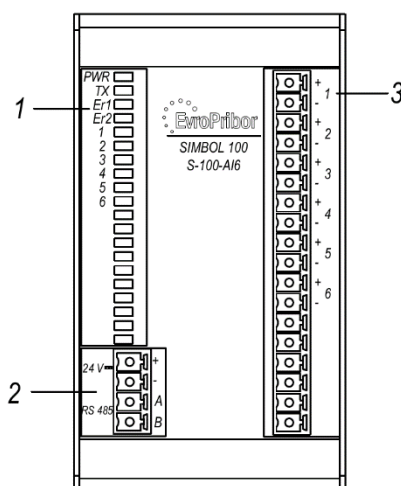
Рисунок 1.2 – Лицевая панель модуля S-100-A16
