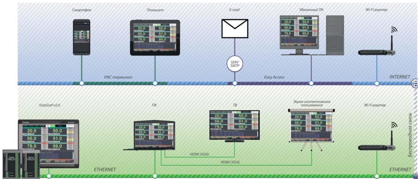
Рис. 5. Схема удаленной работы с комплексом измерительным видеографическим VizoGraf V2.0
